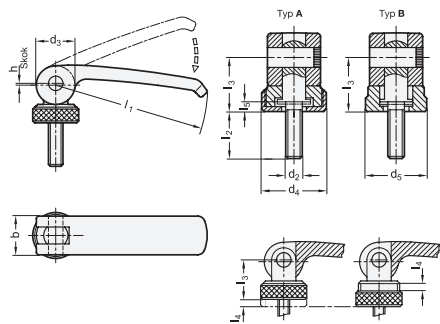
GN 927.7-A-Z trzpieniem gwintowanym, podkładka oporowa ze stali nierdzewnej, z nakrętką regulacyjną STAINLESS STEEL
