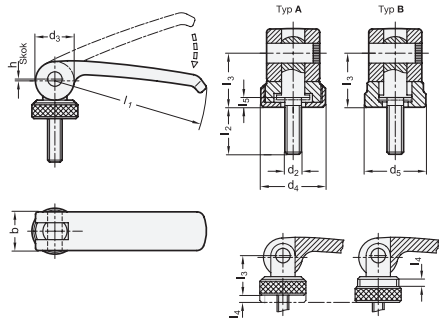
GN 927.7-B-Z trzpieniem gwintowanym, podkładka oporowa ze stali nierdzewnej, bez nakrętki regulacyjnej STAINLESS STEEL
